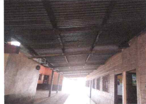
Foto 6. Vista del modulo corredor con vigas de madera, se propone cambiar a estructura de metal y ca,mbiar el techo por lamina troquelada cal 26.
